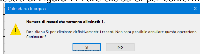
Figura 7 - conferma cancellazione
