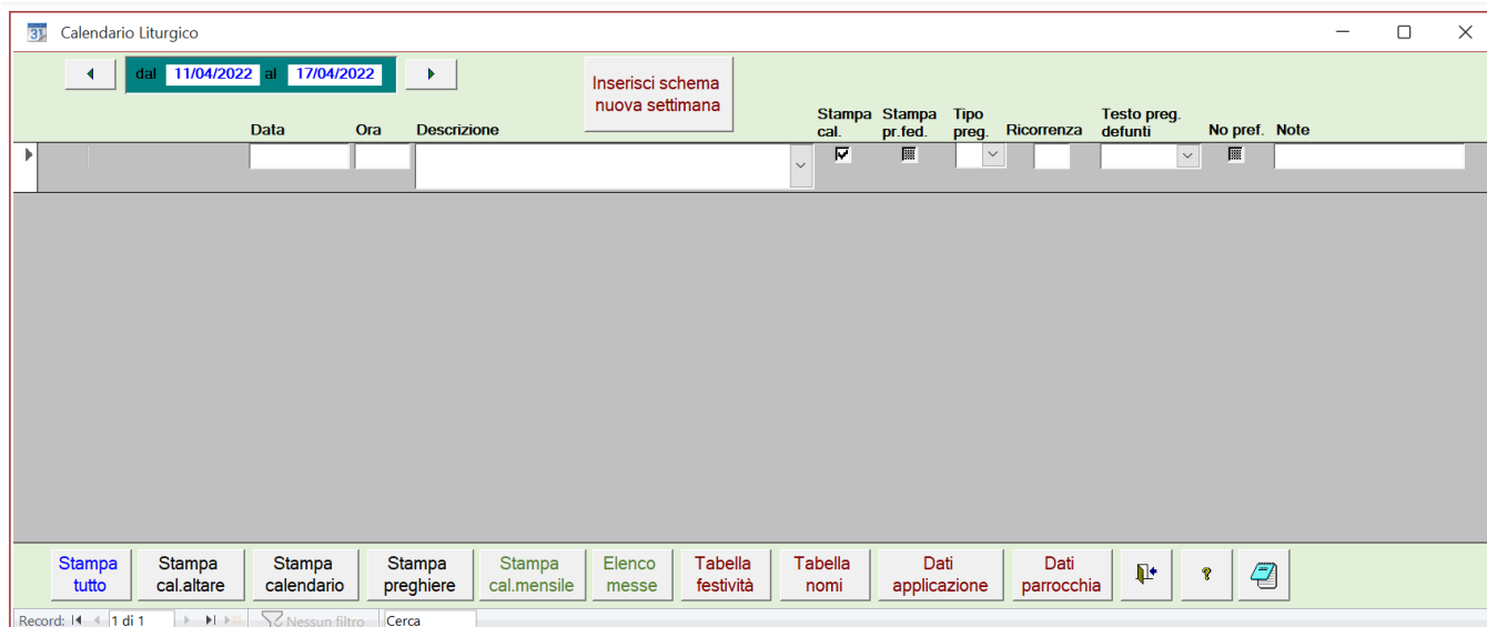
Figura 1 – finestra principale
